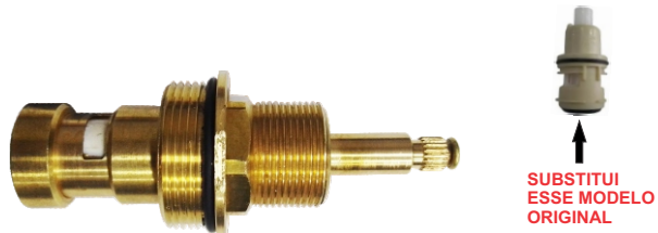
REGISTRO DOCOL BASE TEC 1416 (1/4 VOLTA)
